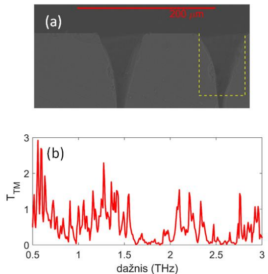
2 pav. Suformuotos periodinės struktūros silicio plokštelėje profilis (a) ir išmatuotas pralaidumo spektras esant TM poliarizacijai (b).
