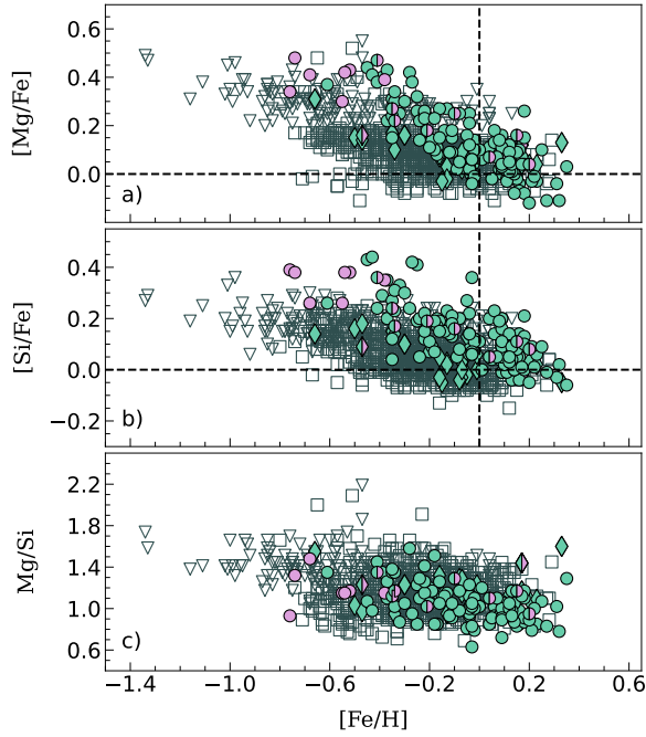
33 pav.: [El/Fe] santykinė magnio ir silicio gausa kartu su Mg/Si santykiu kaip funkcija nuo metalingumo [Fe/H] . Visi simboliai atitinka tokias pat reikšmes kaip ir 32 pav. Duomenys palyginimui (tuščiaviduriai pilki kvadratai plonajam diskui ir trikampiai - storajam diskui) yra paimti iš Mikolaitis et al. (2019) ir Tautvaišienė et al. (2022).
