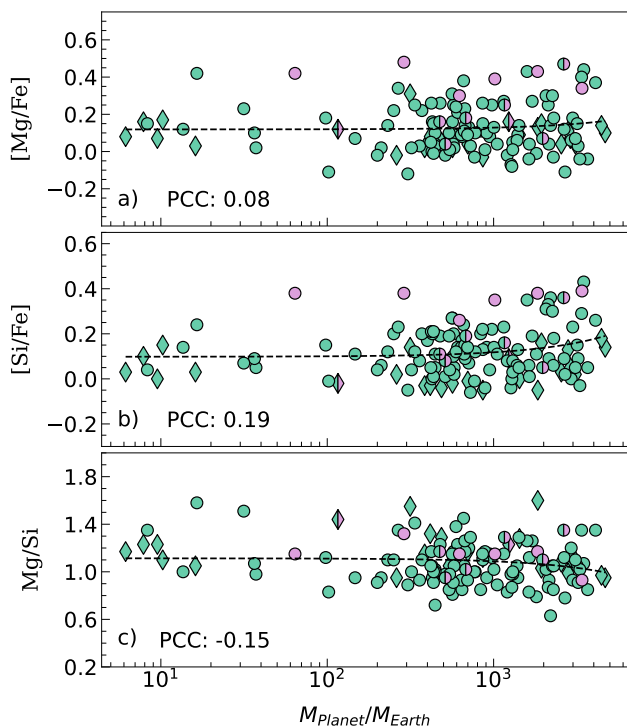
41 pav.: [\text{Mg}/\text{Fe}] , [\text{Si}/\text{Fe}] santykinės gauros ir jų santykis \text{Mg}/\text{Si} pavaizduoti kaip funkcija nuo planetų masių visose tirtose žvaigždėse. Sistemoje esant ne vienai planetai, atsižvelgiama tik į masyviausią planetą. Visi simboliai turi tą pačią reikšmę kaip ir 23 pav.
