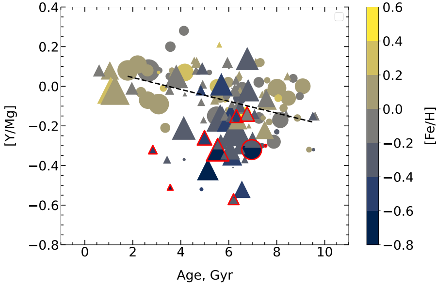
37 pav.: [Y/Mg] NLTE santykis kaip funkcija nuo žvaigždžių amžiaus (miliardais metų, Gyr). Simbolių spalvos pagal [Fe/H] . Visi simboliai turi tą pačią reikšmę kaip ir 36 pav.
