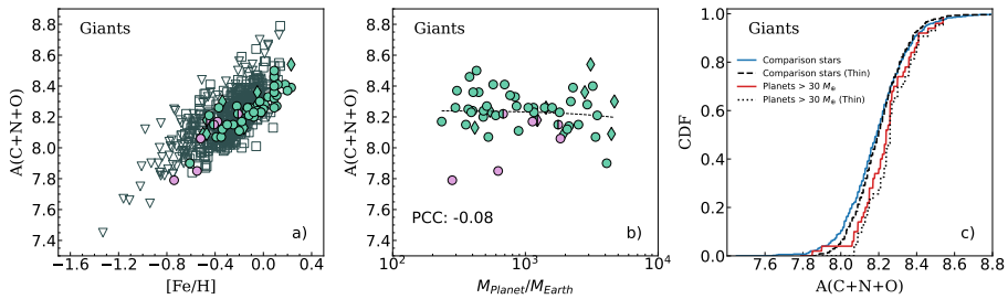
35 pav.: a dalyje: A(C+N+O) gaupos pasiskirstymas [Fe/H] atžvilgiu. b dalyje: ta pati gaupa, priklausomai nuo planetų masių žvaigždės milžinėms. c dalyje: kaupiamasis A(C+N+O) pasiskirstymas žvaigždės milžinėms. Visi simboliai turi tas pačias reikšmes kaip 32 ir 34 pav.
