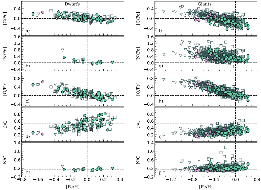
32 pav.: Žvaigždžių su planetomis anglies, azoto ir deguonies santykinė gausa [E/Fe] kartu su C/O ir N/O santykiais kaip funkcija nuo metalingumo [Fe/H] . Kairėje vaizduojami nykštukių rezultatai, dešinėje - milžinių. Plonojo ir storio disko žvaigždės atitinkamai yra pavaizduotos žalia ir rožine spalvomis, o tarpinės, pereinamosios populiacijos žvaigždės pažymėtos spalvotais simboliais. Planetų turinčios žvaigždės iš I Publikacijos yra pavaizduotos rombai. Palyginamosios žvaigždės, neturinčios patvirtintų planetų ir paimtos iš Stonkutė et al. (2020) ir I publikacijos, yra pažymėtos tuščiaviduriais pilkais kvadratais (plonasis diskas) ir trikampaiais (storasis diskas).
