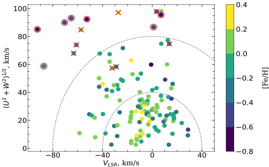
28 pav.: Analizuotų žvaigždžių Toomre diagrama. Simboliai nuspalvinti pagal metalingumą, [Fe/H] . Brūkšninės linijos žymi pastovią suminio erdvinio greičio ( v_{\text{tot}} = (U_{\text{LSR}}^2 + V_{\text{LSR}}^2 + W_{\text{LSR}}^2)^{1/2} ) vertę ties 40 ir 80 \text{km s}^{-1} . Raudonai apibrėžtos žvaigždės priskirtos storio disko populiacijai, o "x" pažymėtos tarpinės plonojo-storio disko žvaigždės.
