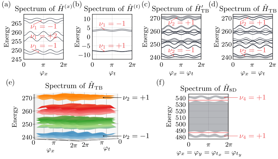
S2 pav.: Sistemų energijos spektrai. (a) Erdvinio hamiltoniano \hat{H}^{(x)} spektras. (b) Laikinio hamiltoniano \hat{H}^{(t)} spektras. (c) Hamiltoniano \hat{H}'_{TB} spektras, lygus Minkovskio sumai spektrų, parodytų (a) ir (b) dalyse. Parodytas spektro pjūvis išilgai linijos \varphi_x = \varphi_t . (d) Hamiltoniano \hat{H}_{TB} energijos spektras išilgai linijos \varphi_x = \varphi_t . (e) Hamiltoniano \hat{H}_{TB} energijos juostos. (f) Aštuonmatės sistemos energijos spektras, gautas sudėjus dvi nepriklausomas 4D sistemas, kurių spektrai parodyti (e) dalyje. Pilki plotai atitinka energijų juostas (atskiri lygmenys nėra parodyti), o raudoni plotai nurodo draustinius tarpus.
