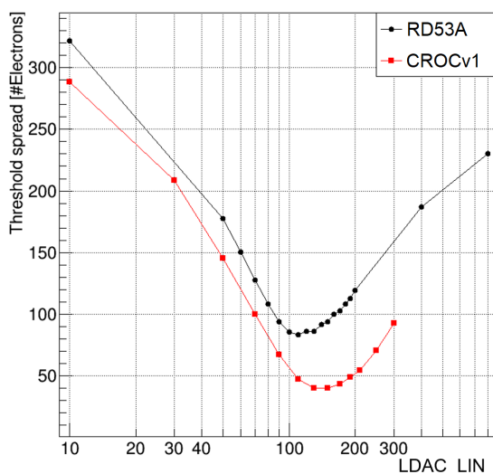
6 pav.: Tipinis RD53A ir CROCV1 lustų signalų aptikimo slenksčių pasiskirstymų standartinių nuokrypių palyginimas esant skirtingoms LDAC registro reikšmėms [A2, B2, B3].
