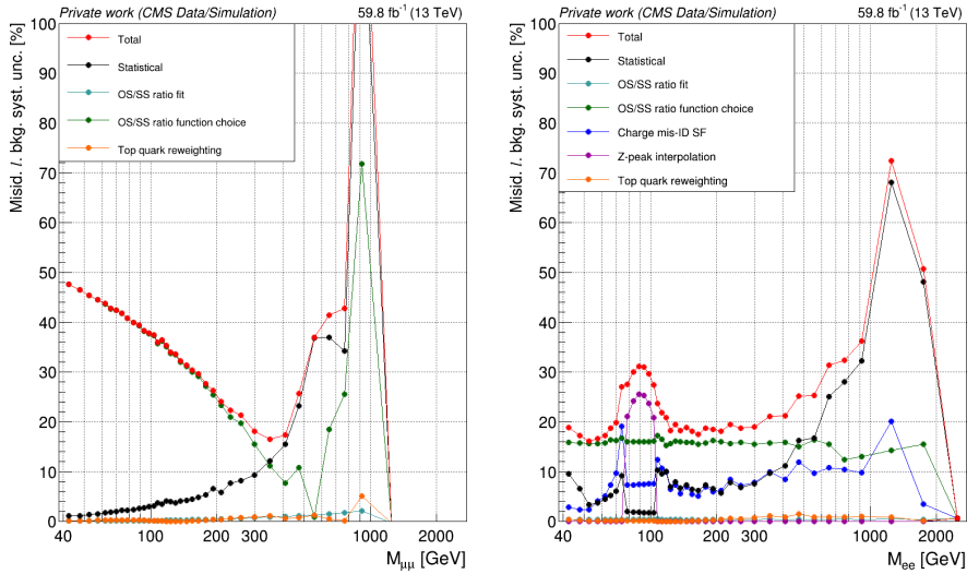
2 pav.: Santykiniai klaidingai atpažintų leptonų fono neapibrėžtumai 2018 m. duomenims miuonų (kairėje) ir elektronų (dešinėje) kanaluose. Kitais duomenų rinkimo laikotarpiais gauti panašūs rezultatai.
