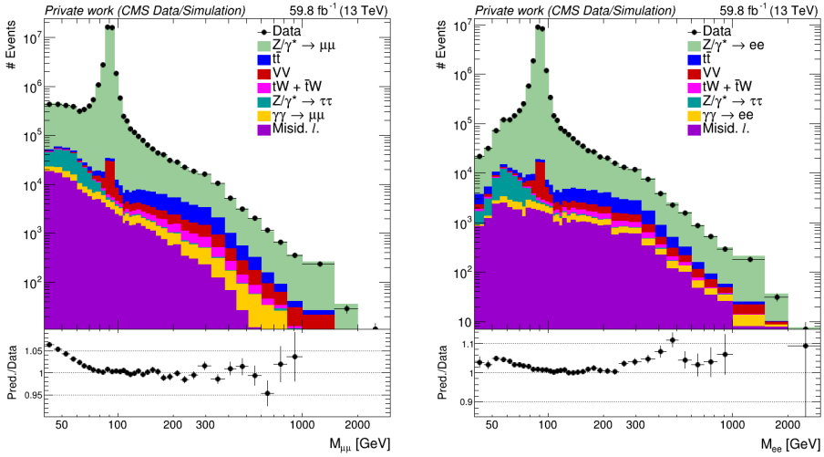
4 pav.: 2018 m. duomenų ir galutinės signalo („ Z/\gamma^* \rightarrow \mu\mu “ arba „ Z/\gamma^* \rightarrow ee “) bei fono prognozės palyginimas miuonų (kairėje) ir elektronų (dešinėje) kanaluose. Kitais duomenų rinkimo laikotarpiais gauti panašūs rezultatai.
