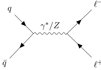
1 pav.: Drell-Yan proceso medžio lygmens Feinmano diagrama.
