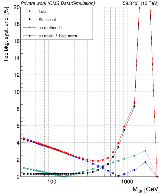
3 pav.: Santykinė e\mu metodu nustatytos viršūninių kvarkų fono pataisos sisteminė neapibrėžtis dimiuonų kanale 2018 m. duomenims. Kitais duomenų rinkimo laikotarpiais gauti panašūs rezultatai.
