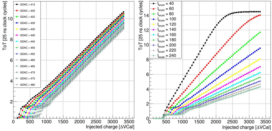
7 pav.: Vidutinė signalo stiprio priklausomybė nuo į pikselį injekuoto krūvio. Kairėje: esant skirtingoms signalo aptikimo slenksčio reikšmėms; dešinėje: esant skirtingoms signalo stiprintuvo grandinės kondensatoriaus iškrovimo srovės reikšmėms [B3].
