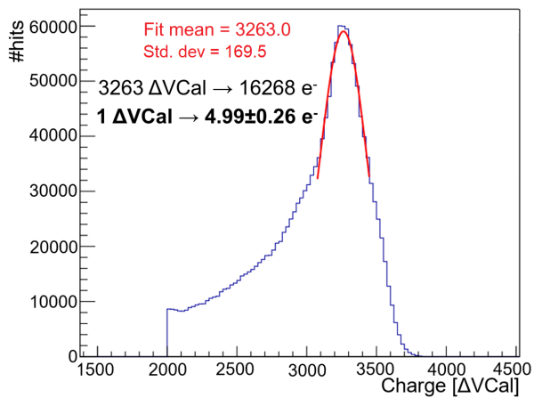
9 pav.: ^{241}\text{Am} rentgeno spindulių detektoriuje sukulto signalo stiprio pasiskirstymas [B3].
