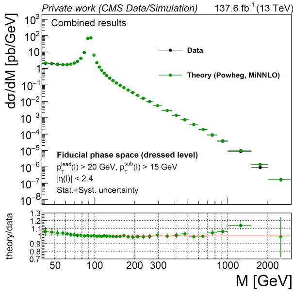
5 pav.: DY diferencialinis reakcijos skerspjūvis d\sigma/dM_{\ell\ell} tiriamojame fazinės erdvės srityje ir jo palyginimas su PowHEG MiNNLO prognoze.
