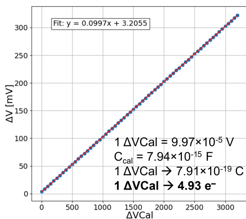
8 pav.: Lusto savikalibracijos grandinės įtampos priklausomybė nuo \Delta V_{\text{Cal}} parametro vertės [B3].
